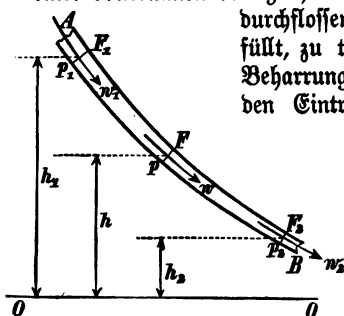
Fig. 27. Bewegung des Wassers in geschlossenem Kanal.
